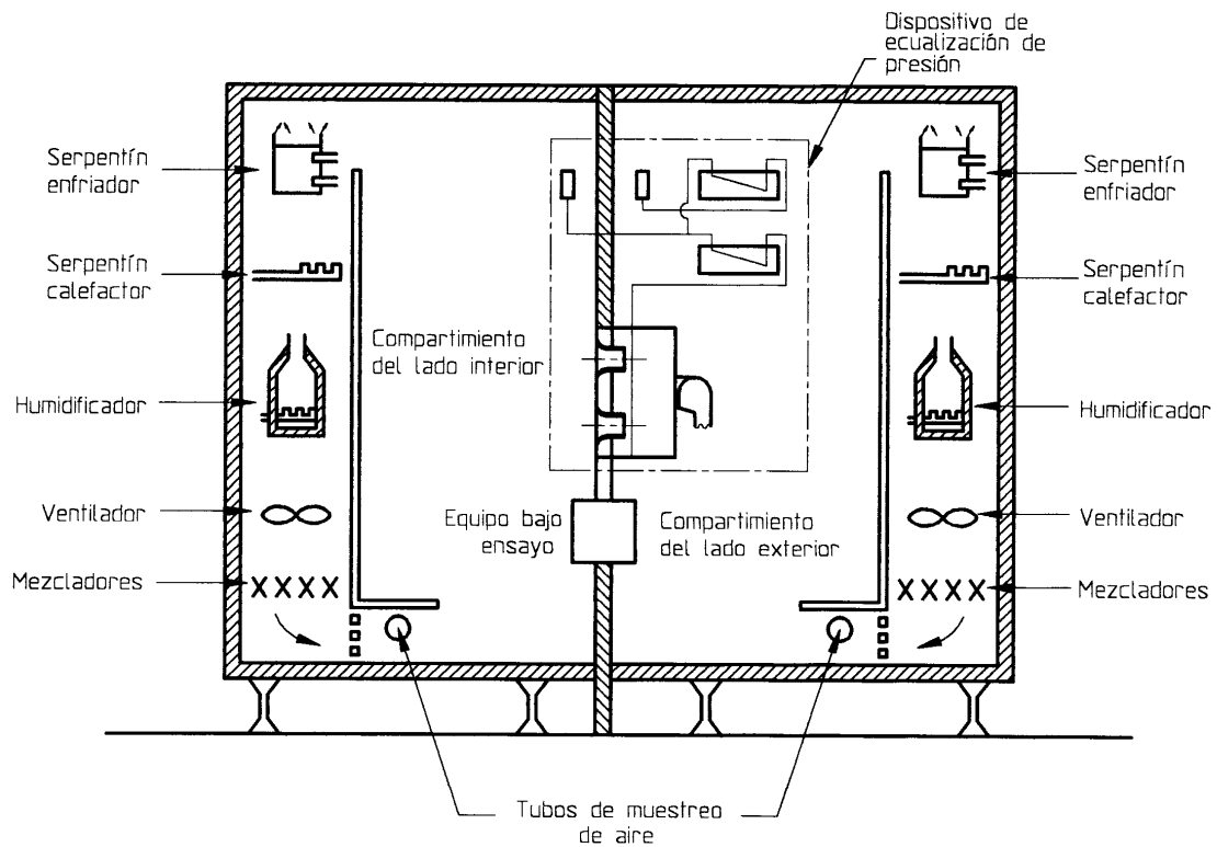
Figura B.4 - Calorímetro tipo sala calibrada típico
