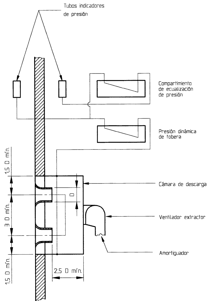
Figura B.1 - Dispositivo de ecualización de presión
