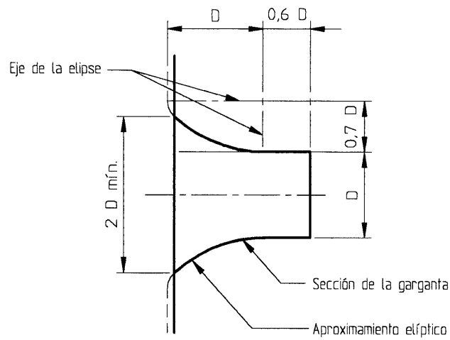
Figura B.2 - Tobera de medición de flujo de aire
