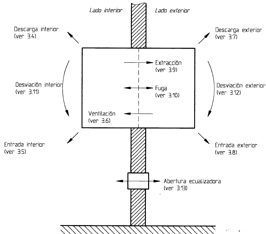
Figura 1 - Diagrama de flujo de aire que ilustra las definiciones dadas en 3.4 a 3.13
