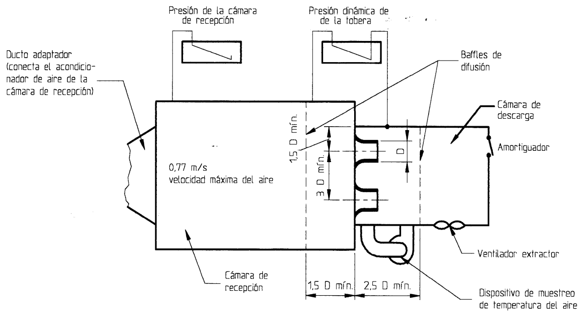
Figura B.3 - Aparato de medición de flujo de aire
